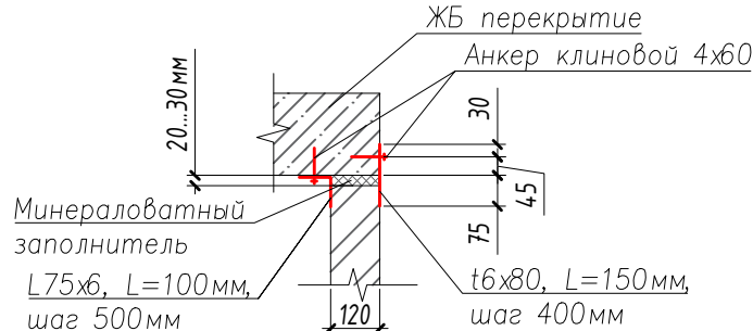
Узел крепления верха существующей перегородки
