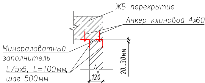
Узел крепления верха заменяемой перегородки
