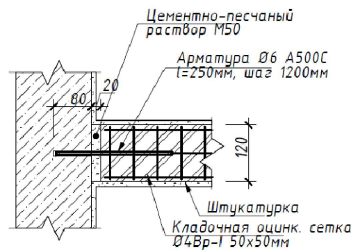
Деталь крепления кирпичной перегородки толщ. 120мм к стенам
